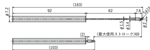
FPD-0760B□-BW(Bタイプ)
