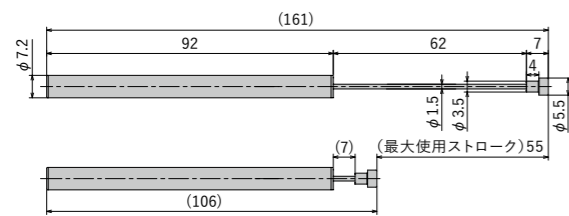
FPD-0760A□-CW(Cタイプ)
