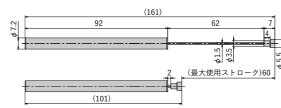
FPD-0760B□-CW(Cタイプ)
